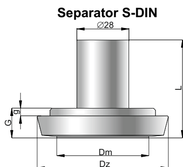
Separatorzy S-DIN zgodnie z DIN11851 dla rur wg DIN 11850 szereg 2
