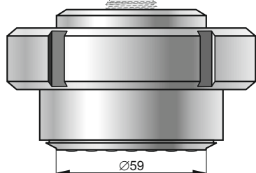
Separator typu S-Poziom 50 mm
