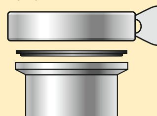
Złącze Tri-Clamp2" z uszczelką i kłamarą
