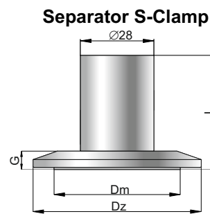
Separatorzy S-Clamp zgodnie z DIN32676 dla rur wg DIN11866 szereg C lub ASME BPE
