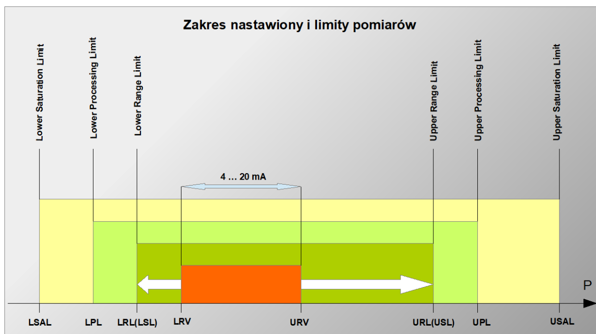
Rysunek 21. Zakres nastawiony i limity pomiarów.
