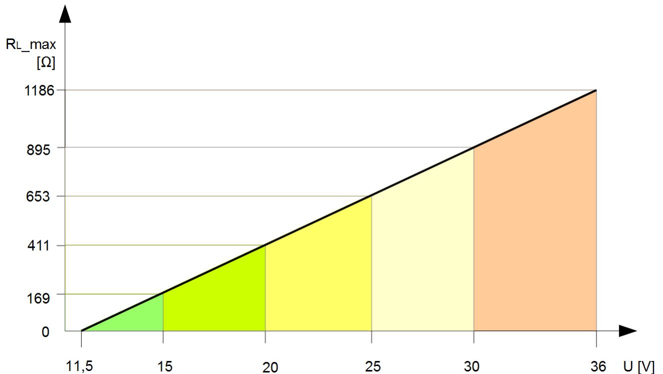
Rysunek 27. Maksymalna rezystancja obciążenia R_{L\_MAX} [ \Omega ] w linii zasilania przetwornika w zależności od napięcia zasilacza U [V].
