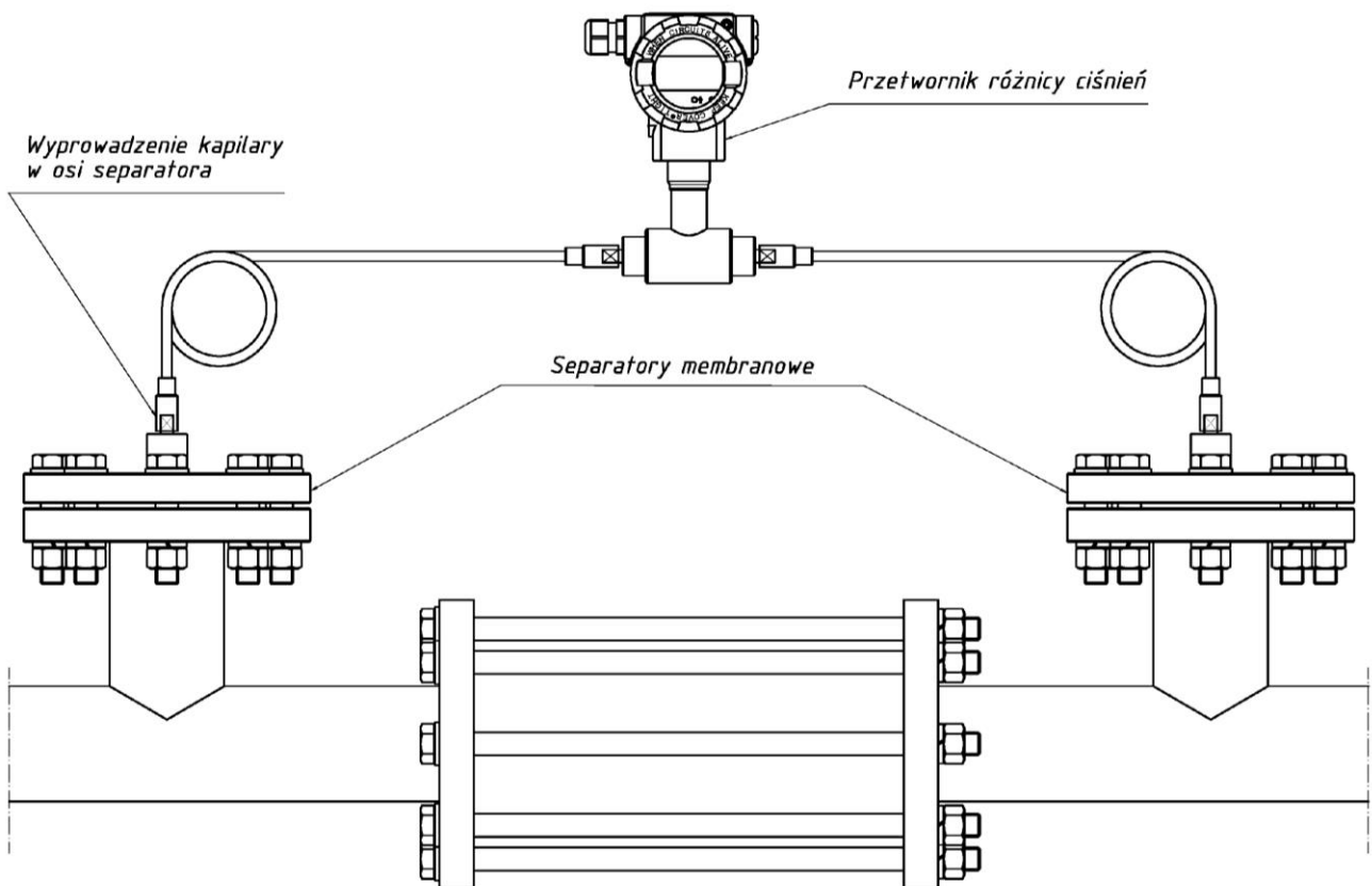
Rysunek 142. Przykład montażu przetwornika APR-2000ALW Safety z separatorami odległościowymi.
