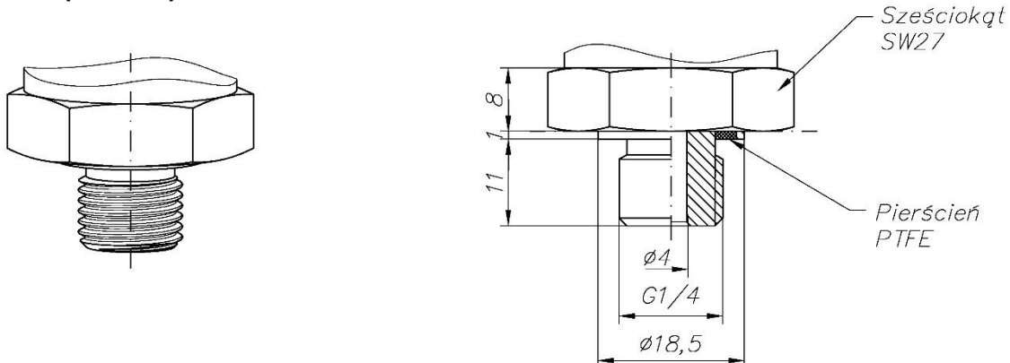
Rysunek 49. Przyłącze G ¼ (G ¼" Ø4).
