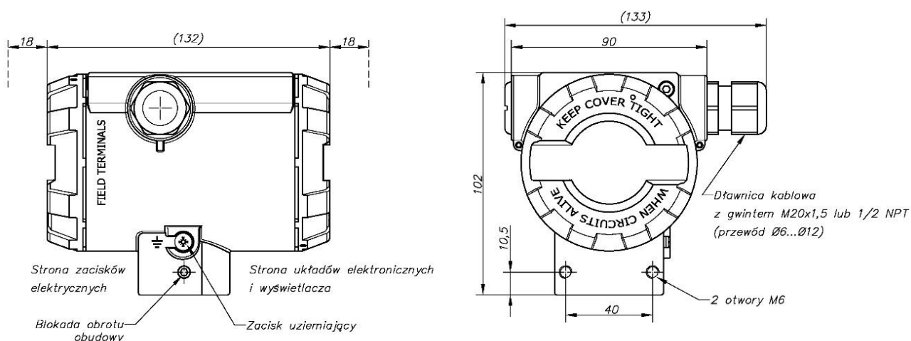
Rysunek 40. Wymiary gabarytowe APC(R)-2000ALW Safety.
