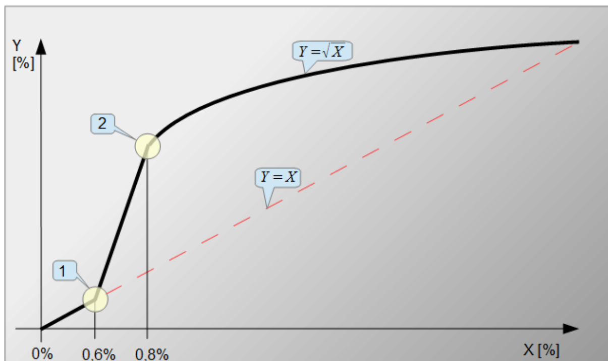
Rysunek 23. Charakterystyka pierwiastkowa "producenta 1" ze stałymi punktami zmiany charakterystyki w punktach 0,6% i 0,8%.
