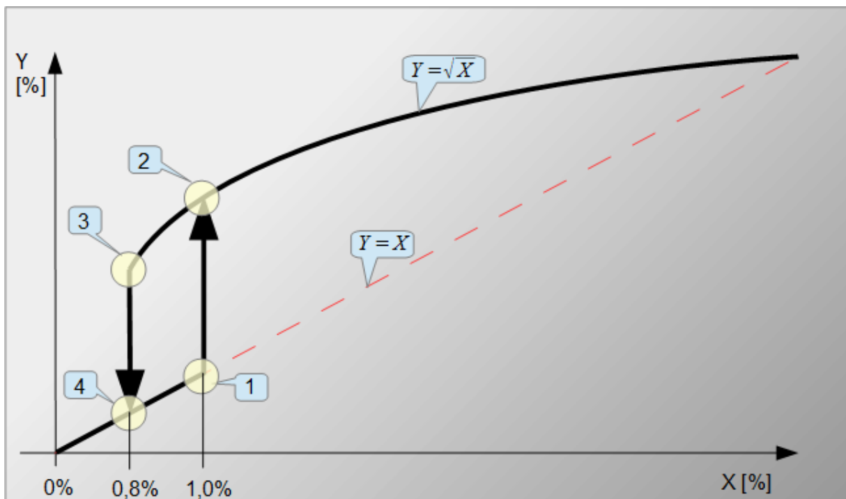
Rysunek 24. Charakterystyka pierwiastkowa "producenta 2" z regulowanym punktem nieczułości i histerezą 0,2%.
