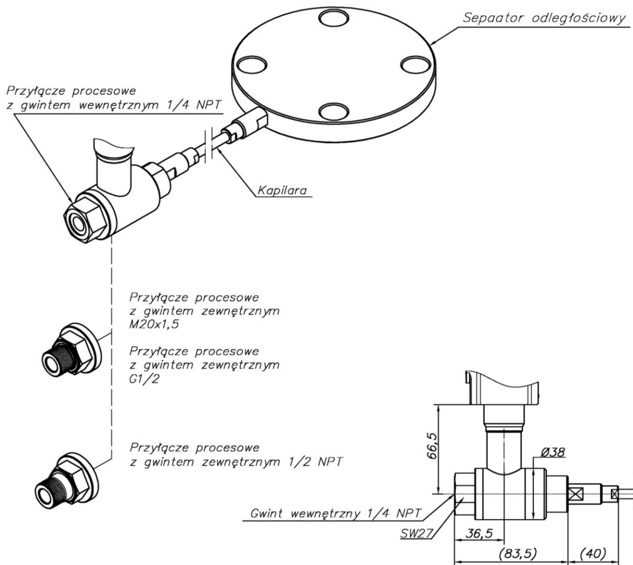
Rysunek 78. Separador odległościowy oraz możliwe do zastosowania przyłącza.
