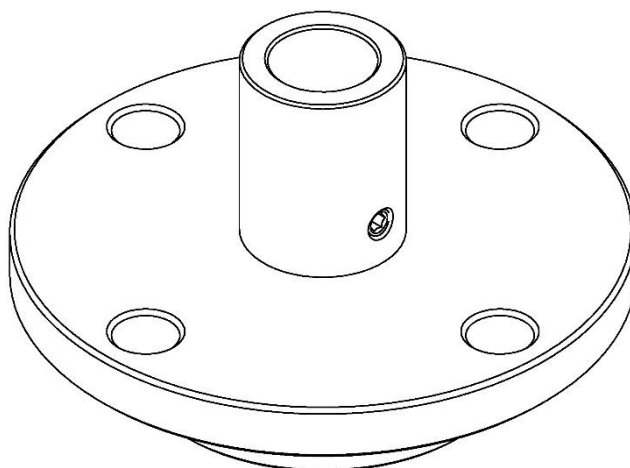
Rysunek 126. Separator S-DRD 65 - widok w izometrii.
