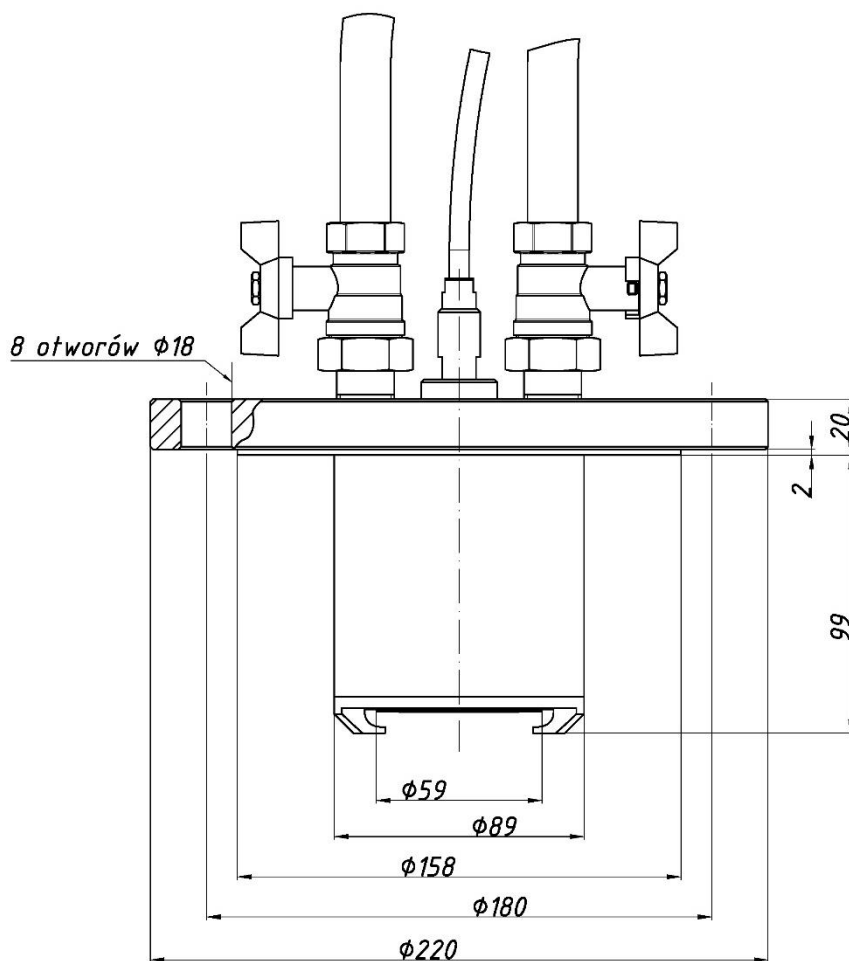
Rysunek 86. Separator S-TK-P z wbudowanym zespołem sfluowania membrany - gabaryty.
