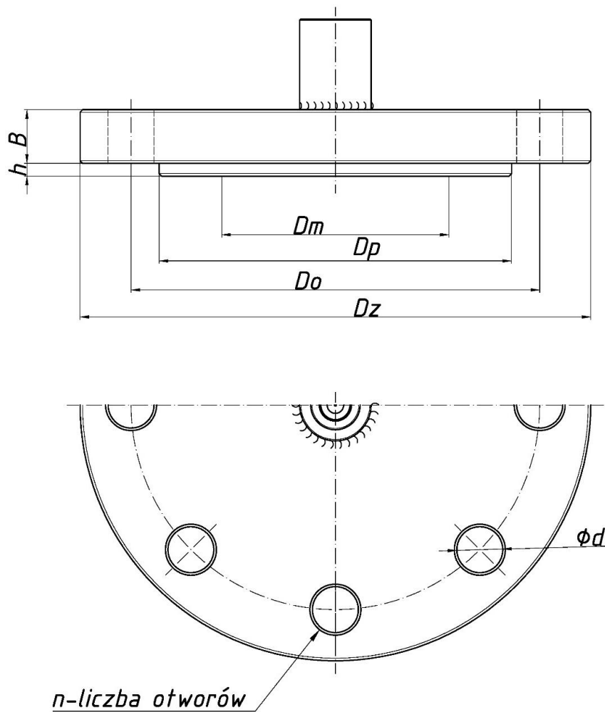
Rysunek 87. Separator kołnierzowy chemoodporny S-Ch.
