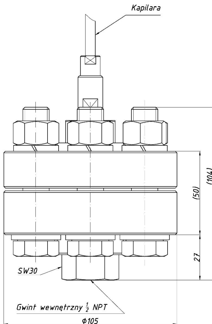
Rysunek 101. Separator S-Comp60MPa - gabaryty.
