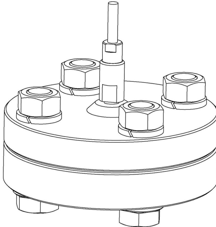
Rysunek 96. Separator S-Comp10MPa - widok w izometrii.
