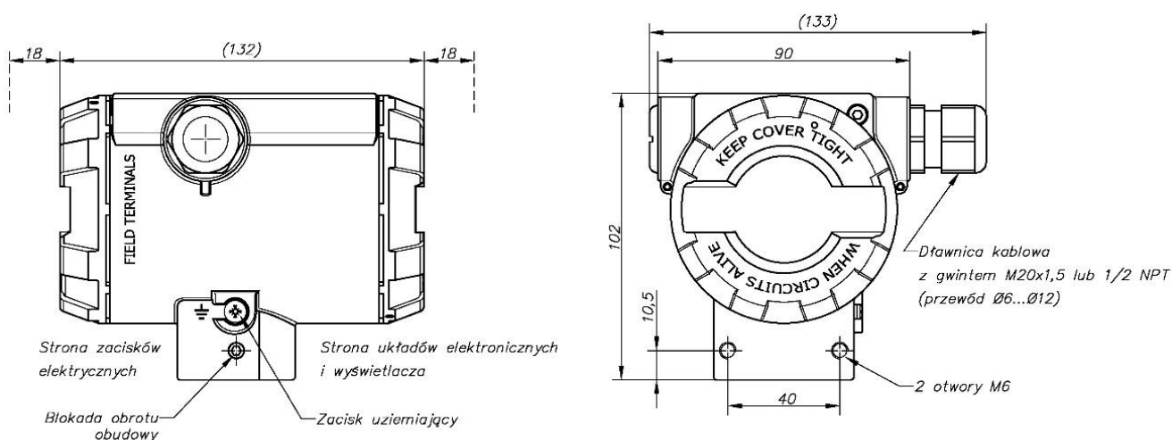
Rysunek 42. Wymiary gabarytowe APC(R)-2000ALW.
