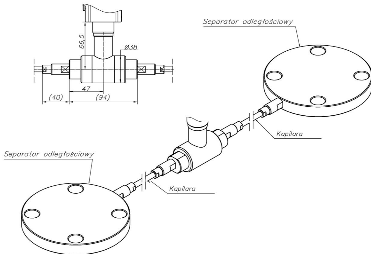
Rysunek 79. Przykład połączenia z wykorzystaniem dwóch separatorów odległościowych.
