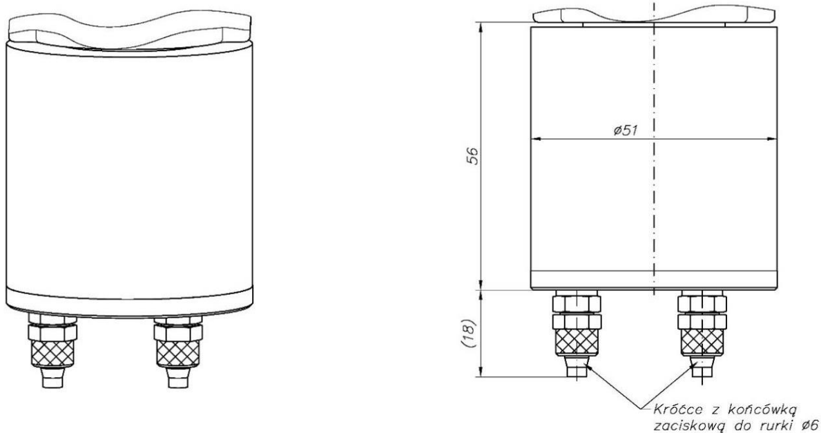
Rysunek 64. Przyłącze procesowe typ PCV.
