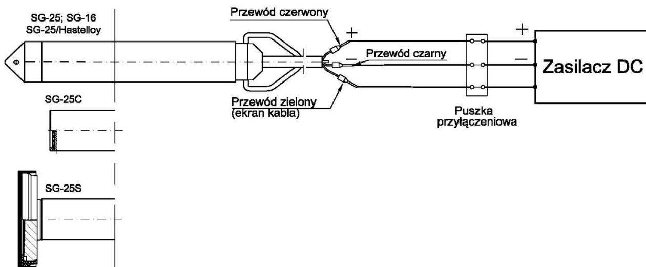
Rysunek 3. Podłączenie elektryczne sondy w wykonaniu standardowym.
