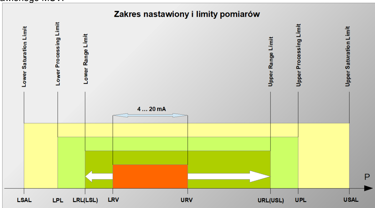
Rysunek 5. Zakres nastawiony i limity pomiarów
