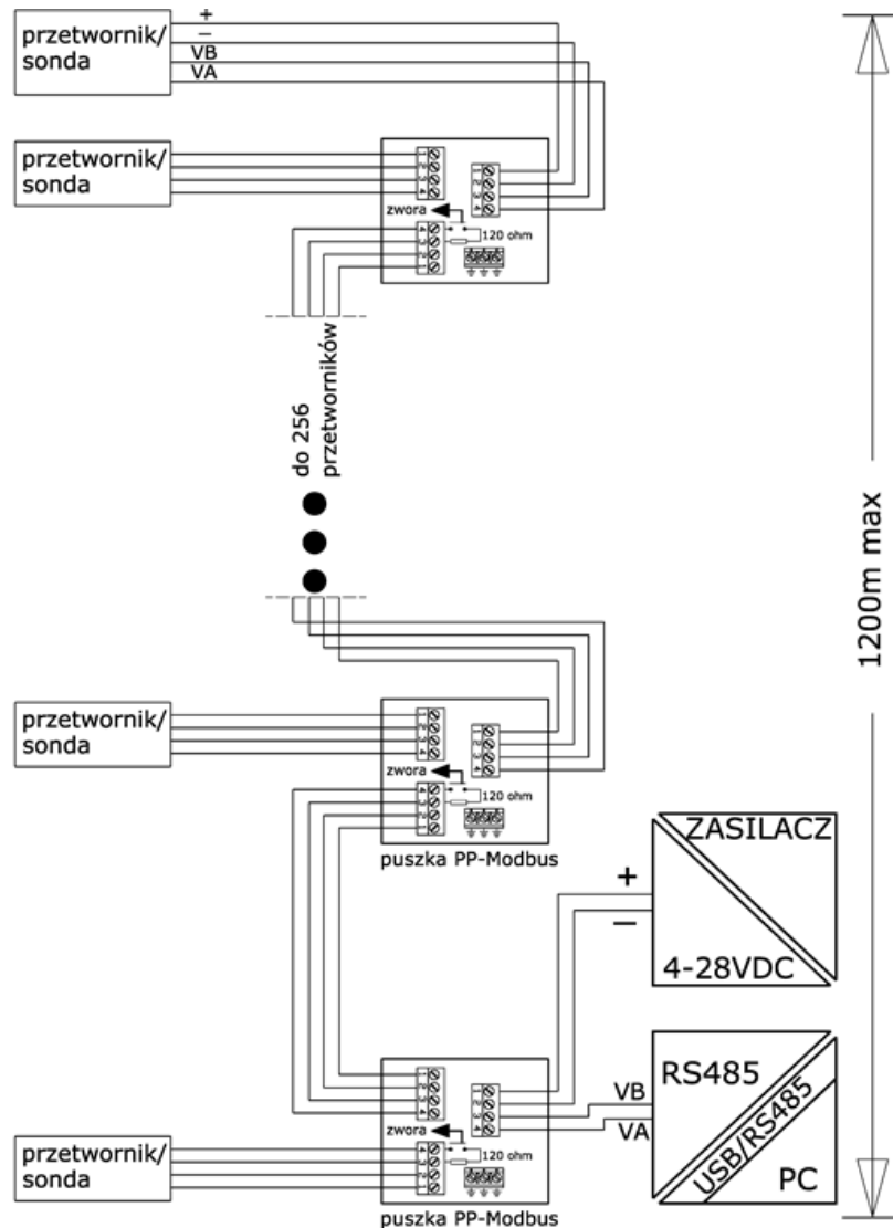
Rysunek 3. Połączenia w sieci Modbus
