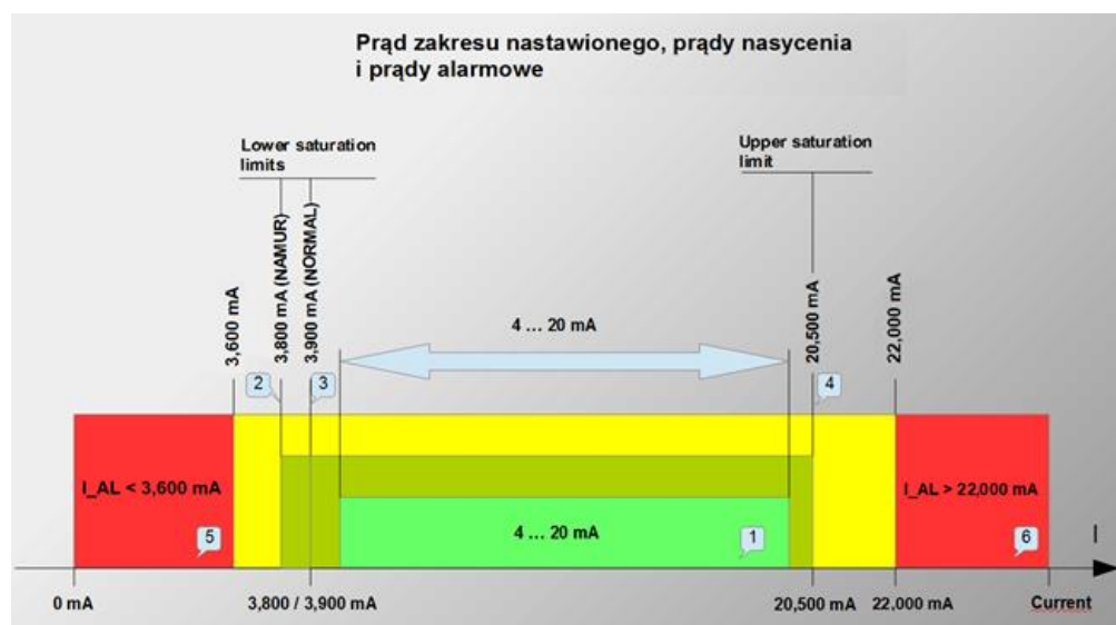
Rysunek 3. Prąd zakresu nastawionego, prądy nasycenia, prądy alarmowe przetworników w wersji standardowej Exi
