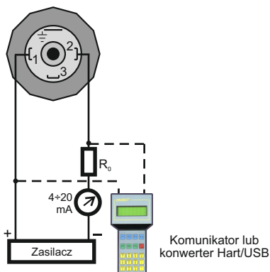
Przyłącze typu PD
