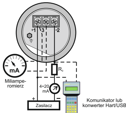
Przyłącze typu PZ
