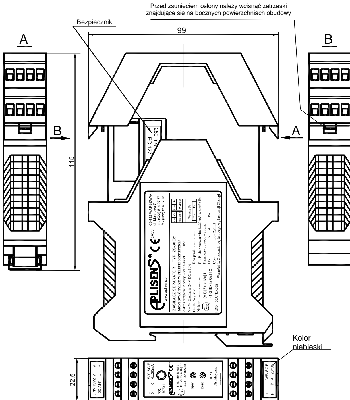
Rys.5. Zasilacz separator ZS-30Ex1 w obudowie listwowej.
