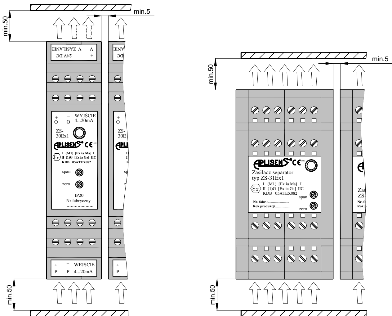
Rys.2. Sposób montażu zasilaczy-separatorów ZS-30Ex1, ZS-31Ex1
