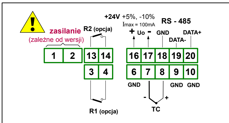
Rys. 4.5. Opis wyprowadzeń dla wersji z wyjściami przekaźnikowymi
