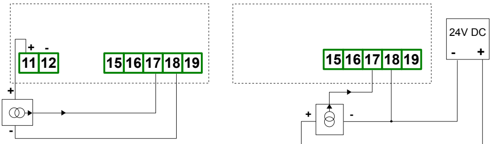
Rys. 4.9. Podłączenia przetworników prądowych 3 przewodowych
