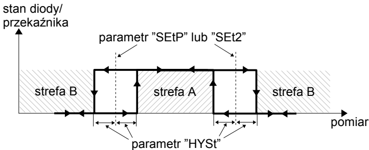
Rys. 6.4. Sterowanie jednoprogowe wyjścia przekaźnikowego/ diody LED
