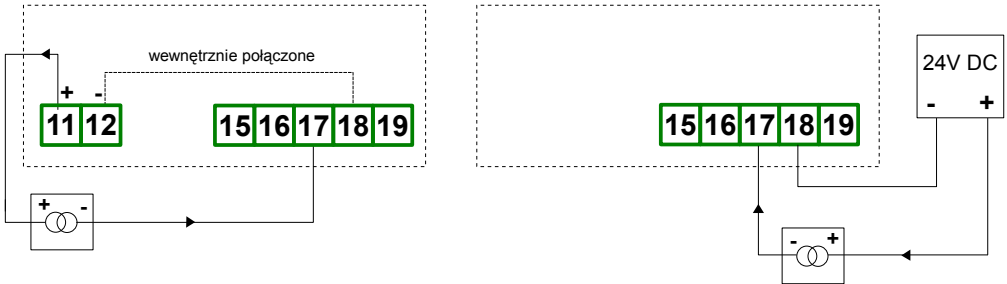
Rys. 4.8. Podłączenia przetworników prądowych 2 przewodowych
