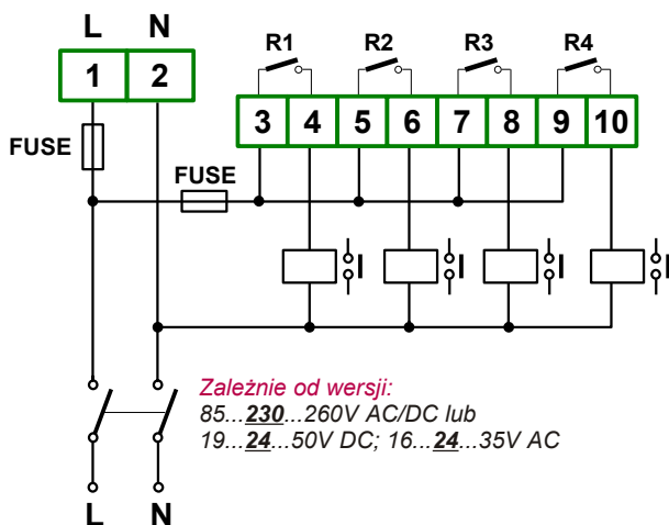
Rys. 4.11. Podłączenie zasilania oraz przekaźników sterujących obciążeniami
