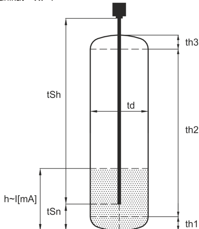
Rys. 12.1 Parametry zbiornika w pozycji pionowej.
