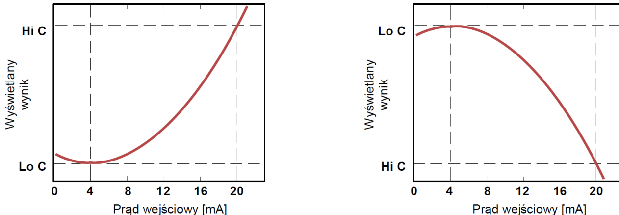
Rys. 13.2 Charakterystyka prosta („Lo C” < ”Hi C”) i odwrócona („Lo C” > ”Hi C”)
