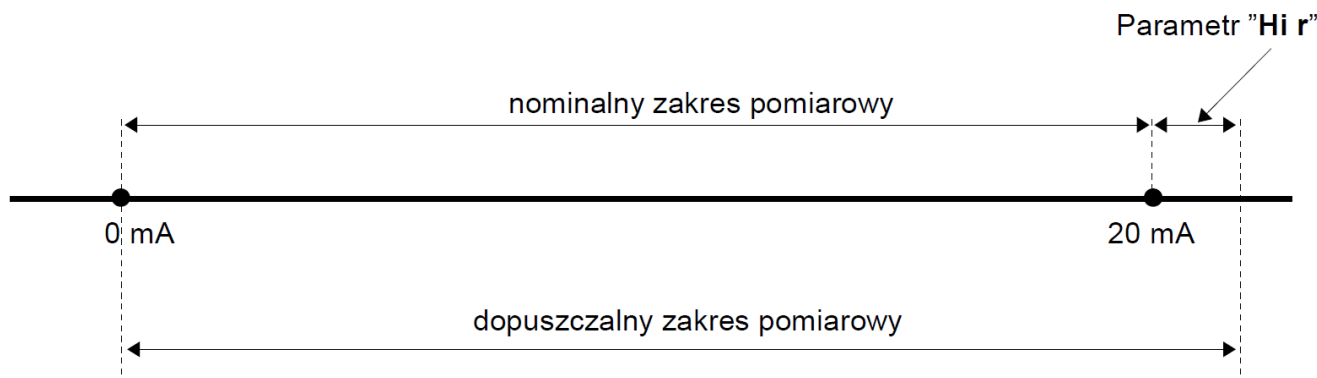
Rys. 11.2 Definicja zakresów pomiarowych w trybie 0 ÷ 20mA
