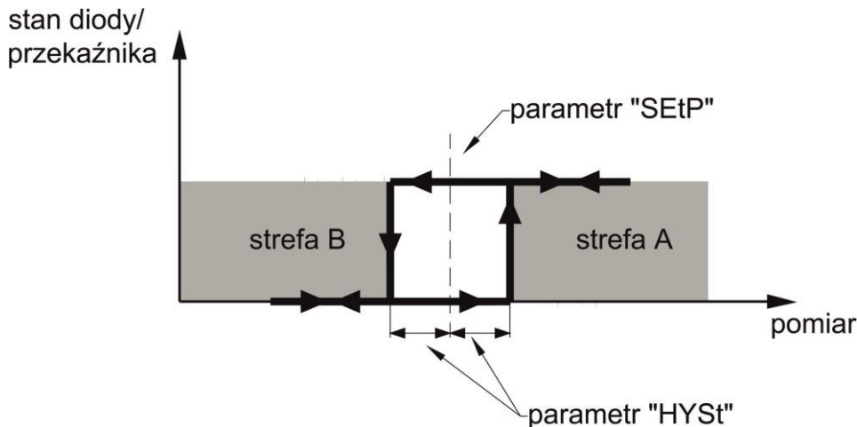
Rys. 11.4 Sterowanie jednoprogowe wyjścia przekaźnikowego/diody LED
