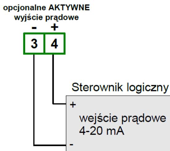
Rys. 8.17 Przykład podłączenia wyjścia prądowego (tylko dla urządzeń posiadających wyjście prądowe)
