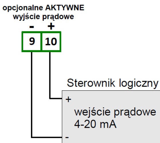
Rys. 8.16 Przykład podłączenia wyjścia prądowego (tylko dla urządzeń posiadających wejście prądowe) – wersja OW
