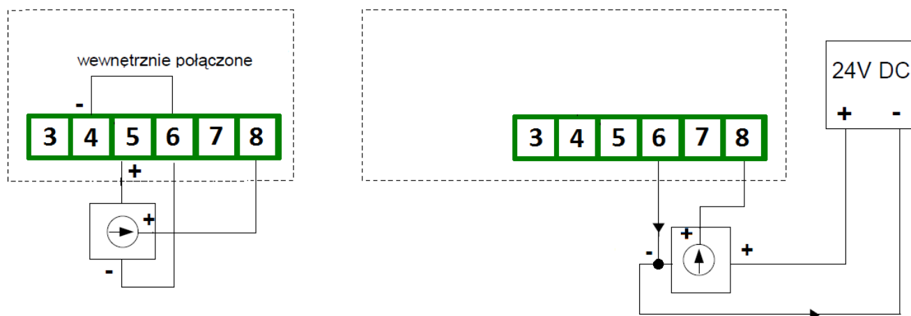
Rys. 8.10 Podłączenia przetworników napięciowych OW
