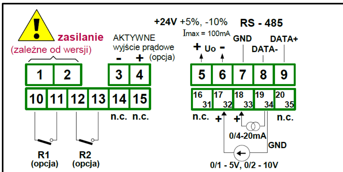
Rys. 8.5 Opis wyprowadzeń dla wersji z dodatkowym aktywnym wyjściem prądowym
