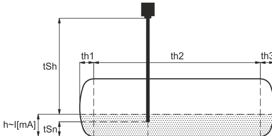
Rys. 12.2 Parametry zbiornika w pozycji poziomej.
