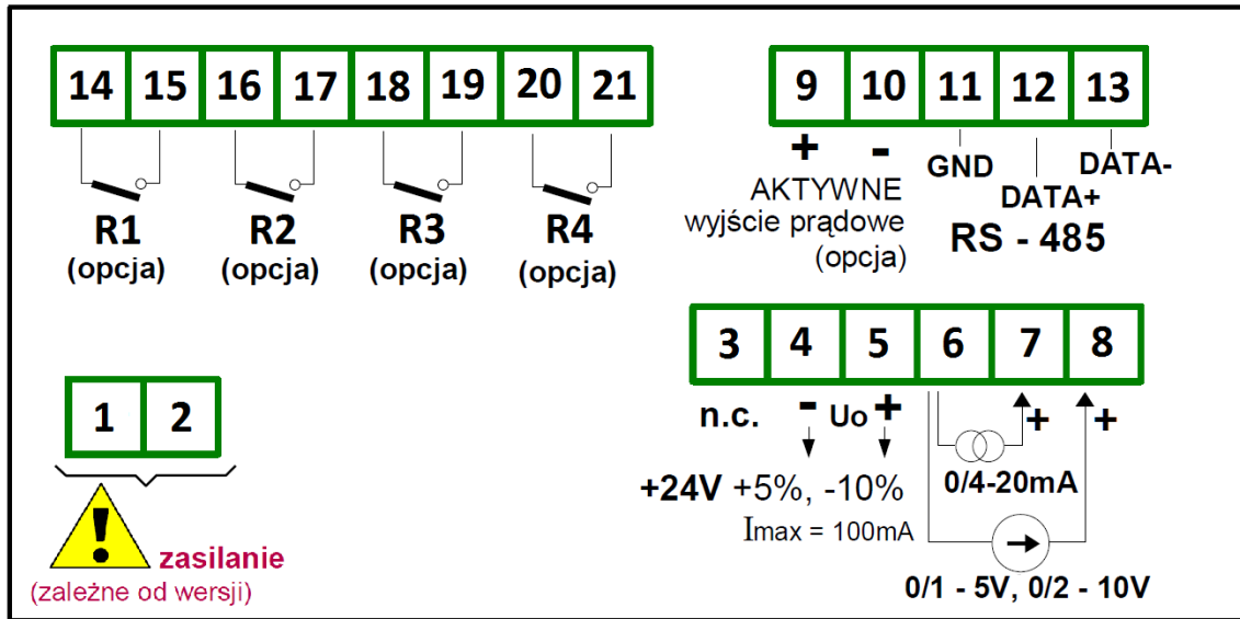
Rys. 8.4 Opis wyprowadzeń dla wersji z dodatkowym aktywnym wyjściem prądowym OW (patrz tabliczka znamionowa)
