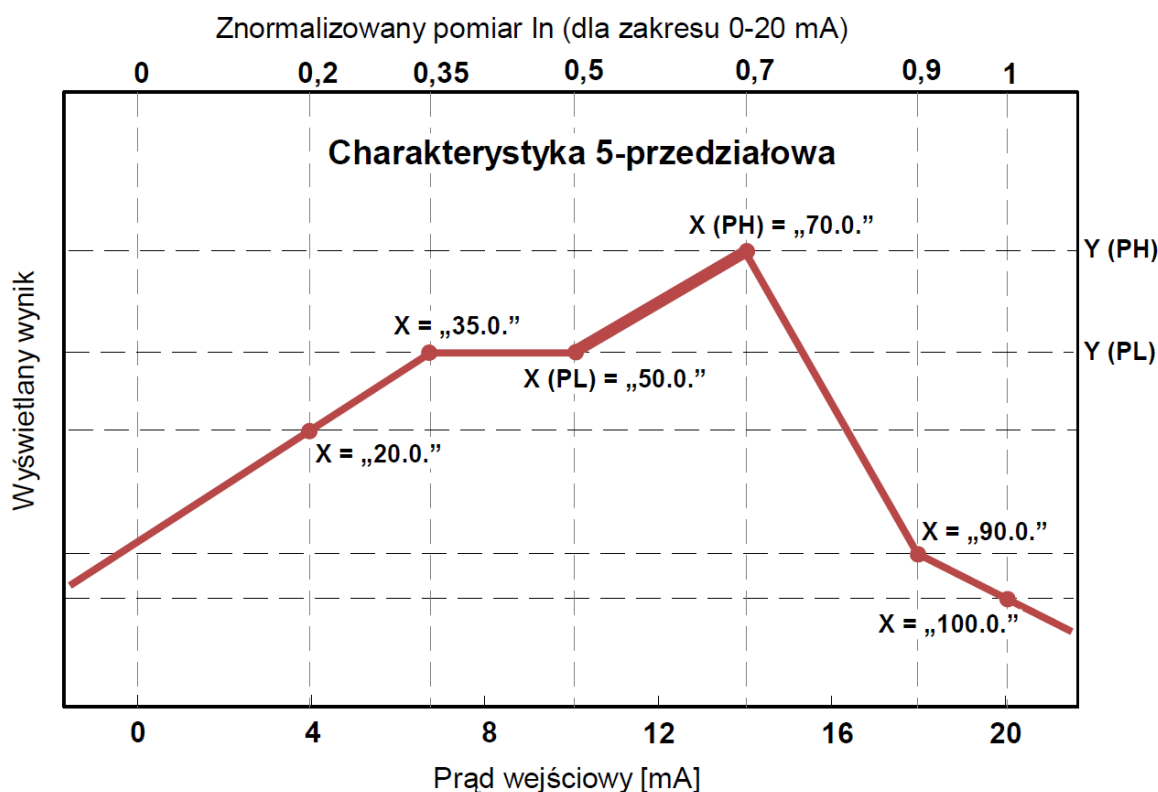
Rys. 13.4 Przykładowa charakterystyka użytkownika
