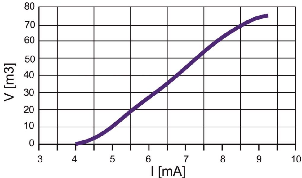
Rys. 13.7 Charakterystyka objętości zbiornika w zależności od prądu wejściowego z sondy poziomoj cieczy w zbiorniku (dla zakresu 4÷20mA).
