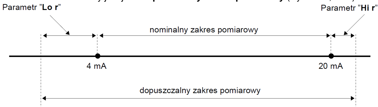
Rys. 11.1 Definicja zakresów pomiarowych w trybie 4 ÷ 20mA
