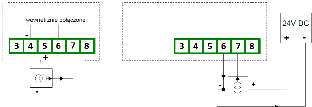
Rys. 8.8 Podłączenia przetworników prądowych 3 przewodowych OW
