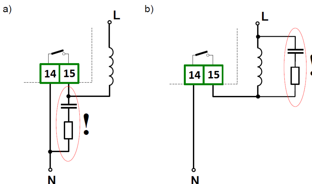
Rys. 8.14 Przykłady równoległego podłączenia obwodu tłumiącego – wersja OW: a) do styków przekaźnika; b) do obciążenia indukcyjnego
