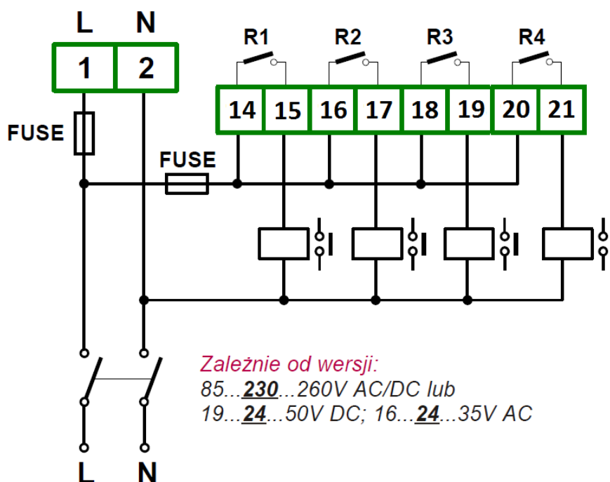
Rys. 8.12 Podłączenie zasilania oraz przekaźników sterujących obciążeniami –wersja OW
