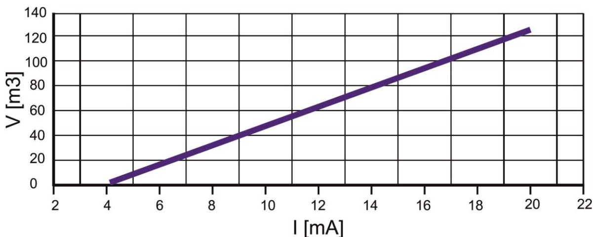
Rys. 13.6 Charakterystyka objętości zbiornika w zależności od prądu wejściowego z sondy poziomej cieczy w zbiorniku (dla zakresu 4÷20mA).
