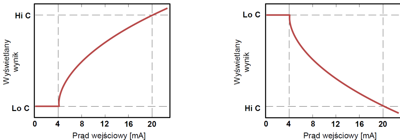
Rys. 13.3. Charakterystyka prosta („Lo C” < „Hi C”) i odwrócona („Lo C” > „Hi C”)
