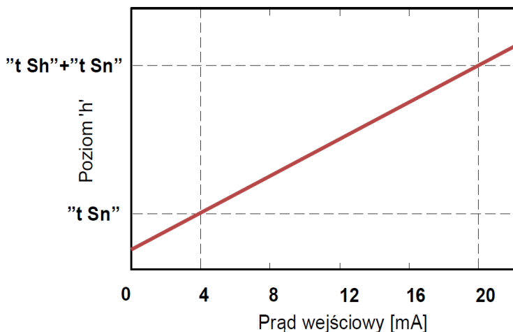
Rys. 13.5 Charakterystyka poziomu cieczy, gazów lub materiałów sypkich w zbiorniku w zależności od prądu wejściowego w zakresie 4-20mA
