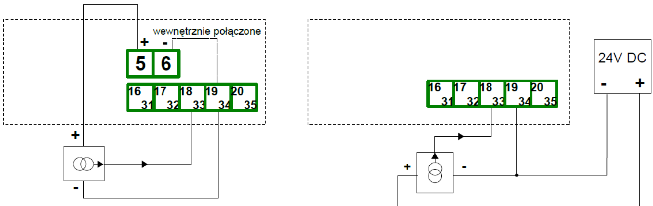
Rys. 8.9 Podłączenia przetworników prądowych 3 przewodowych
