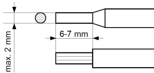
Rys. 8.1 Sposób odizolowania przewodów oraz wymiary końcówek kablowych
