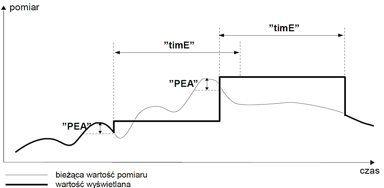
Rys. 11.3 Sposób detekcji wartości szczytowych
