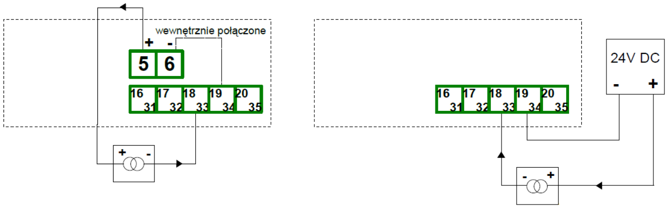
Rys. 8.7 Podłączenia przetworników prądowych 2 przewodowych
