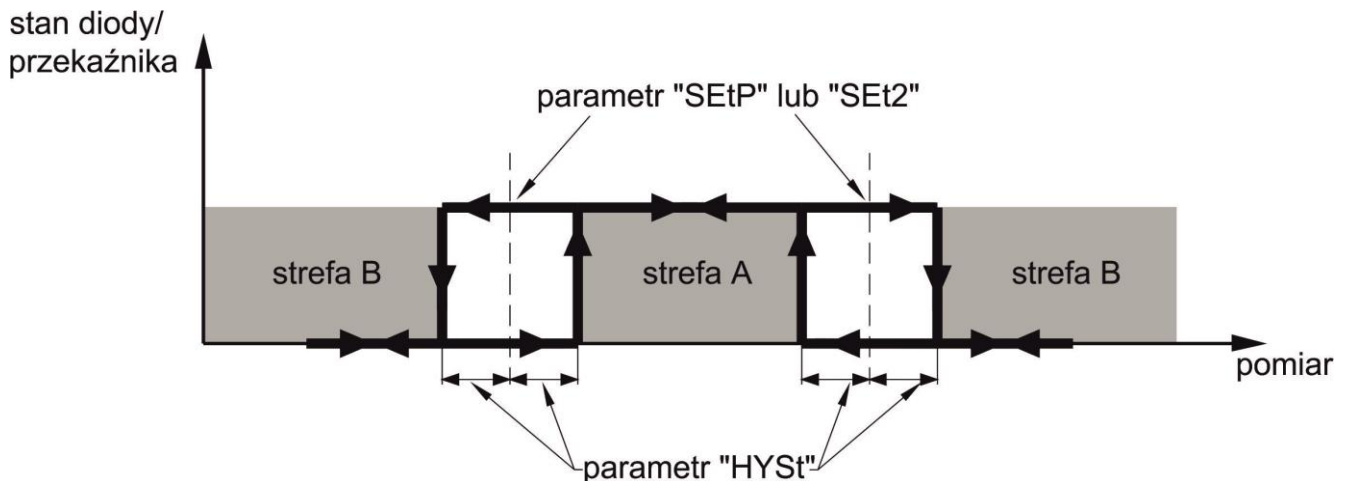
Rys. 11.5 Sterowanie dwuprogowe wyjścia przekaźnikowego/diody LED
