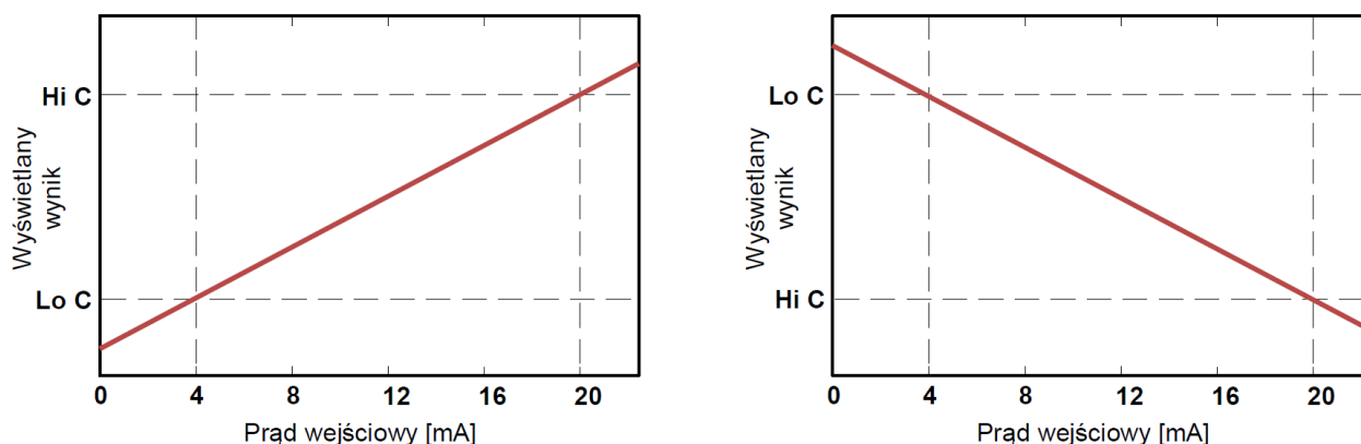
Rys. 13.1 Charakterystyka prosta („Lo C” < ”Hi C”) i odwrócona („Lo C” > ”Hi C”) KONFIGURACJA
