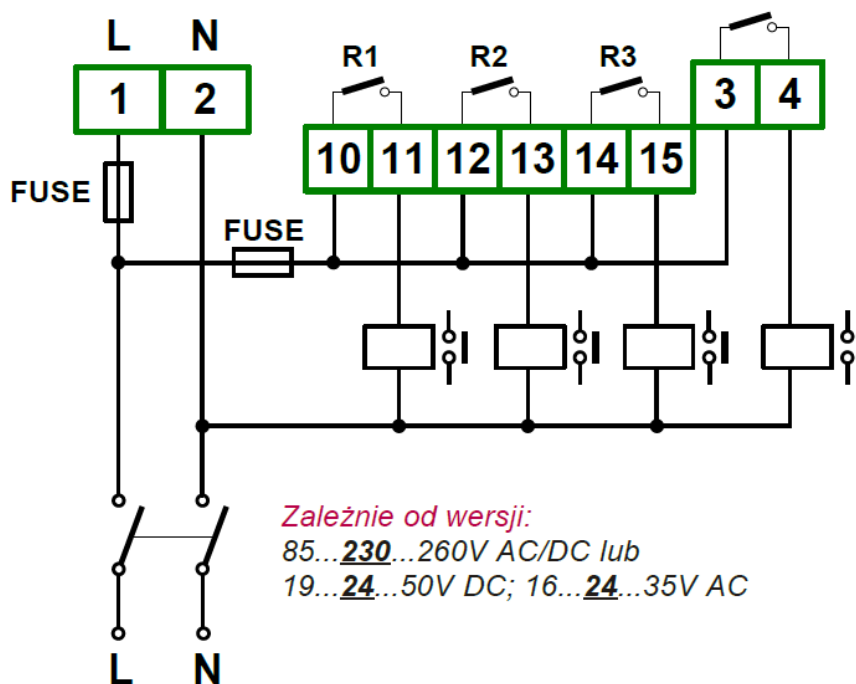
8.13 Podłączenie zasilania oraz przekaźników sterujących obciążeniami
