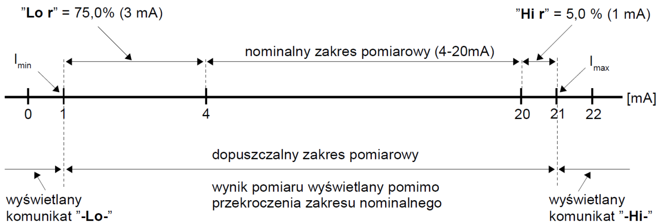
Rys. 12.3 Określenie dopuszczalnego zakresu pomiarowego dla przykładowego ustawienia parametrów "Lo r" i "Hi r" (w trybie "4-20" )
