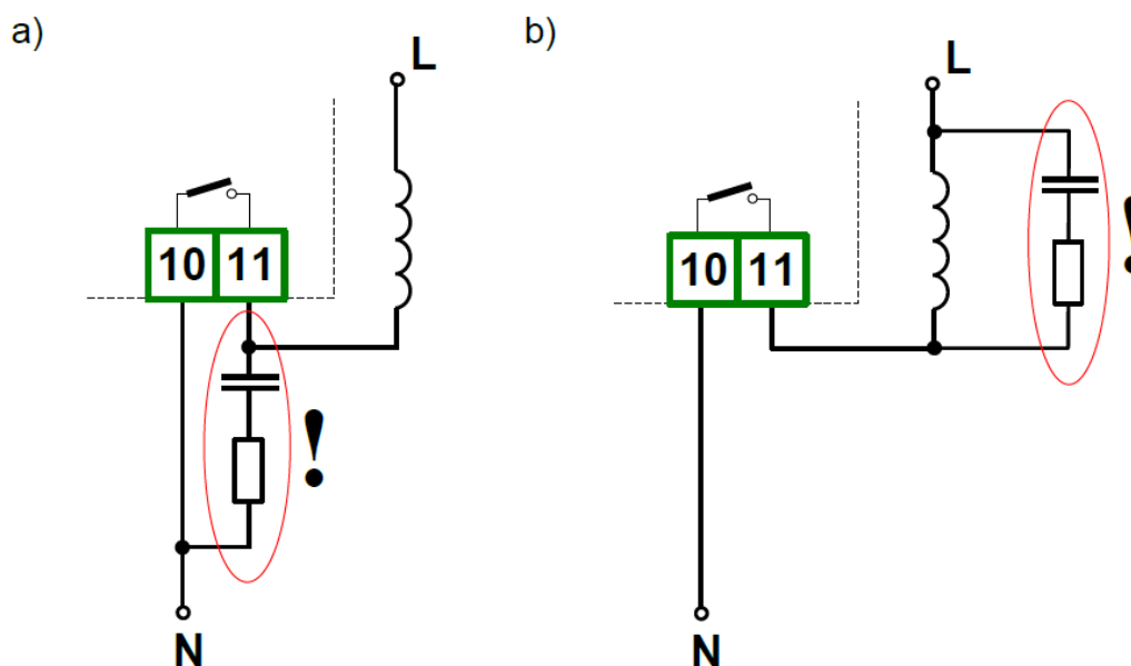
Rys. 8.15 Przykłady równoległego podłączenia obwodu tłumiącego: a) do styków przekaźnika; b) do obciążenia indukcyjnego
