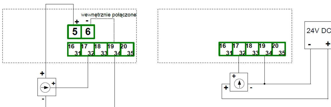
Rys. 8.11 Podłączenia przetworników napięciowych
