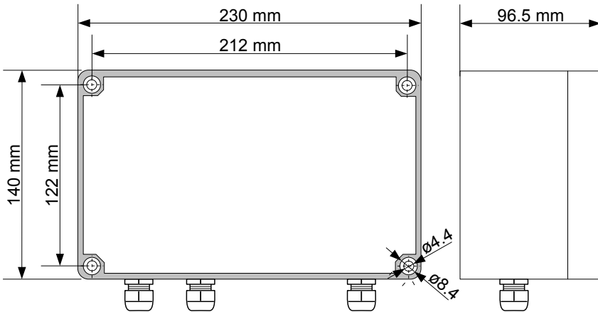
Rys. 4.2. Wymiary montażowe obudowy typu T
