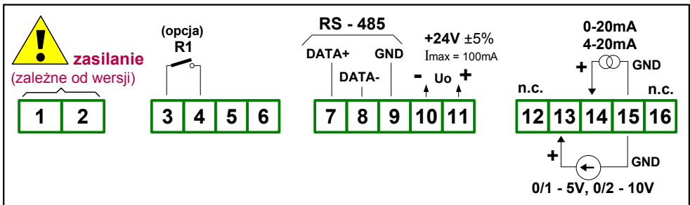
Rys. 4.4. Opis wyprowadzeń dla wersji z wyjściami przekaźnikowymi
