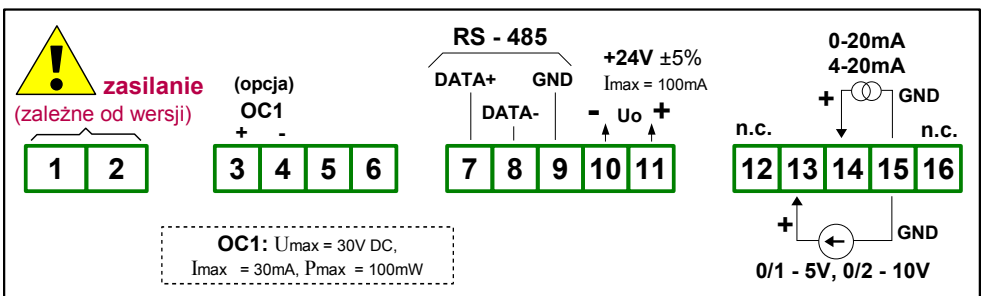
Rys. 4.5. Opis wyprowadzeń dla wersji z wyjściami OC
