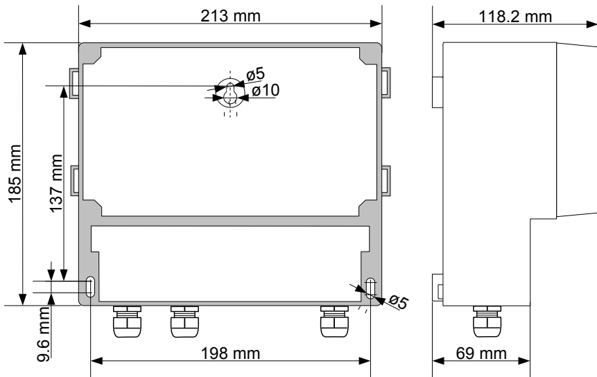
Rys. 4.1. Wymiary montażowe obudowy typu F
