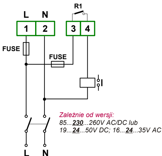
Rys. 4.9. Podłączenie zasilania oraz przekaźnika sterującego obciążeniem
