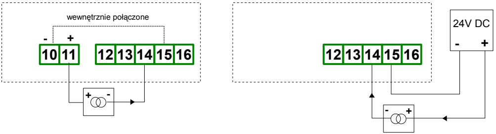
Rys. 4.6. Podłączenia przetworników prądowych 2 przewodowych
