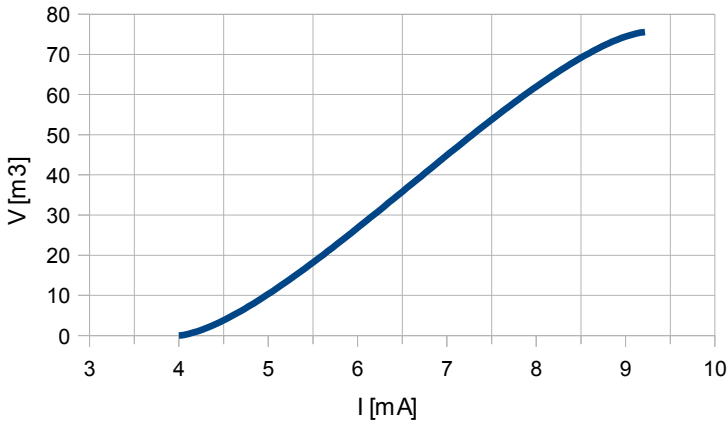
Rys. 9.7 Charakterystyka objętości zbiornika w zależności od prądu wejściowego z sondy poziomego cieczy w zbiorniku (dla zakresu 4÷20mA).
