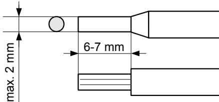
Rys. 4.3. Sposób odizolowania przewodów oraz wymiary końcówek kablowych
