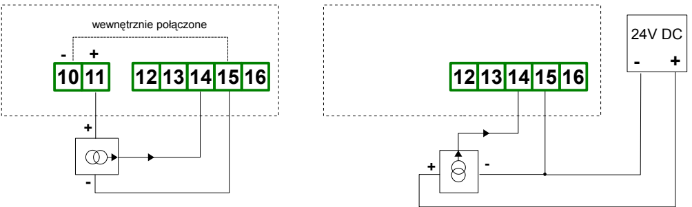
Rys. 4.7. Podłączenia przetworników prądowych 3 przewodowych
