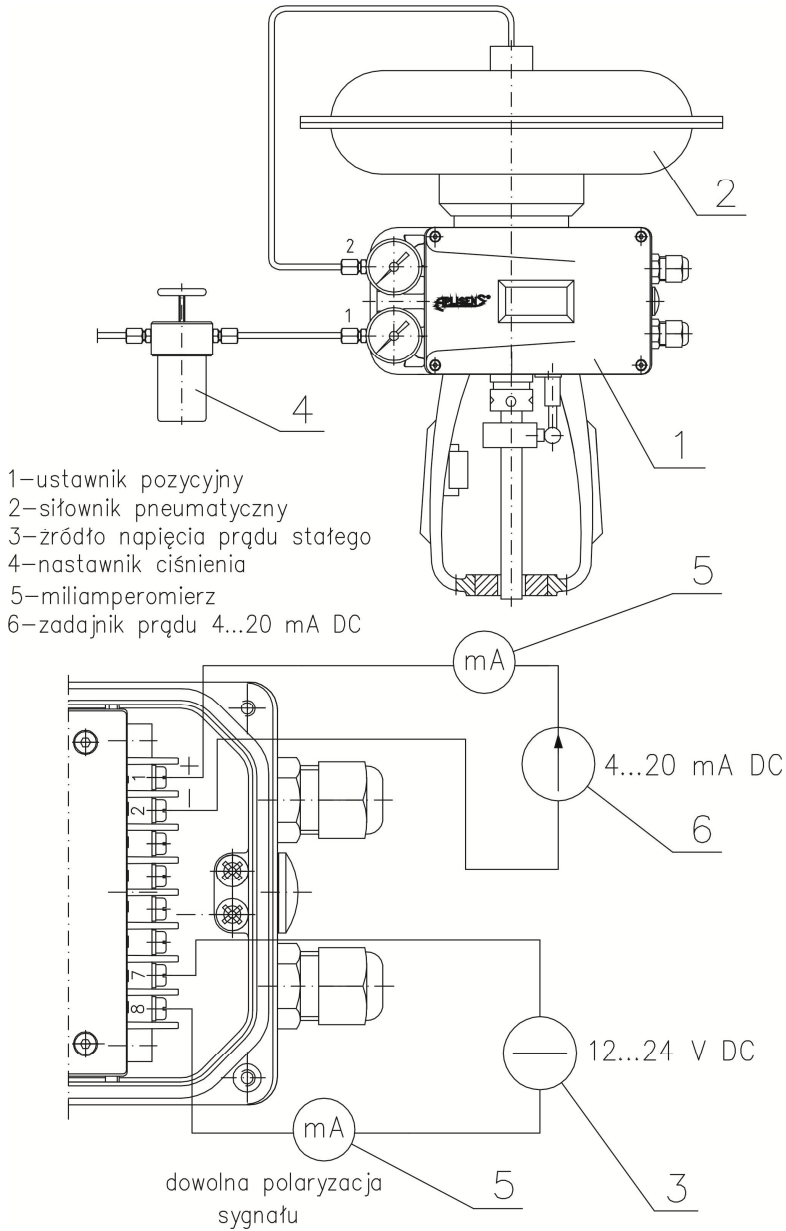
Rys. 17. Schemat układu pomiarowego do uruchomienia ustawnika APIS-1X0-....
