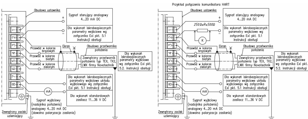
Rys.21d Schemat połączeń elektrycznych ustawnika dla wykonaw z zewnętrznym przetwornikiem położenia w warunkach gdy:
