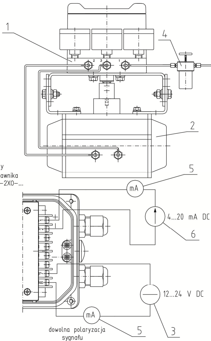
Rys. 18. Schemat układu pomiarowego do uruchomienia ustawnika APIS-1X0-... i APIS-2X0-... (siłownik obrotowy jednostronnego i dwustronnego działania)
