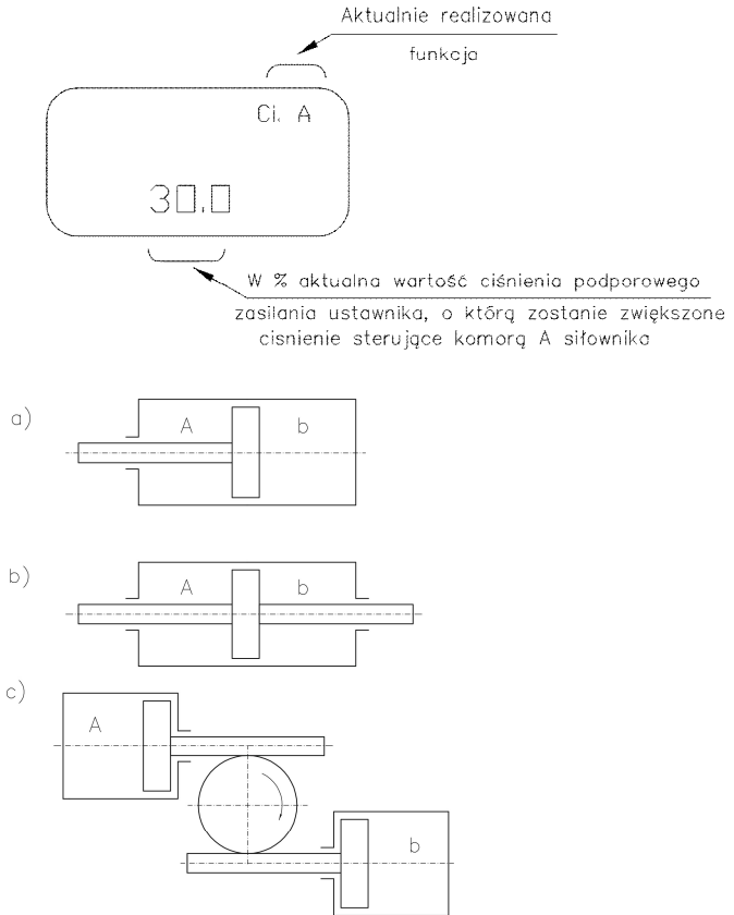
Rys.16. Identyfikacja komór podporowych siłowników dwustronnego działania
