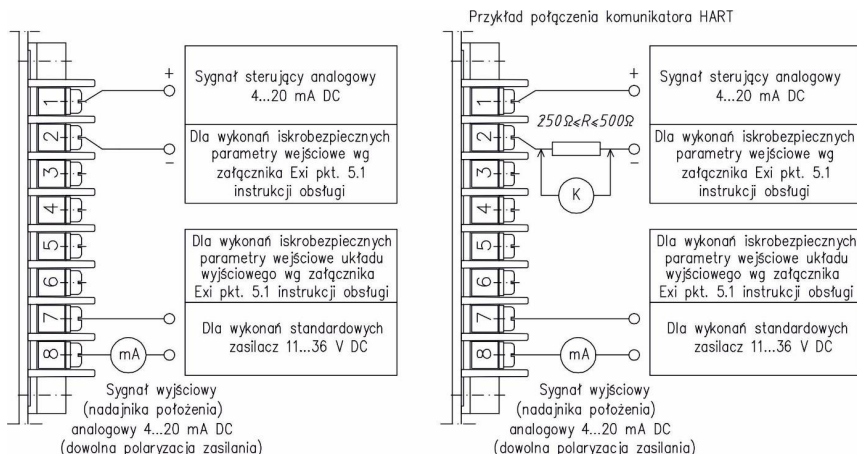
Rys. 21a Schemat połączeń elektrycznych ustawnika dla wykonaw z wewnętrznym przetwornikiem położenia
