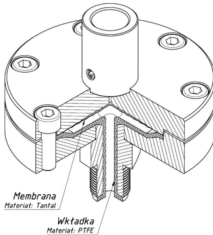
Rysunek 101. Separator S-CompCh - widok w półprzekroju.
