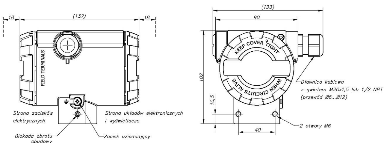
Rysunek 40. Wymiary gabarytowe APC(R)-2000ALW Exd, Exi/Exd.
