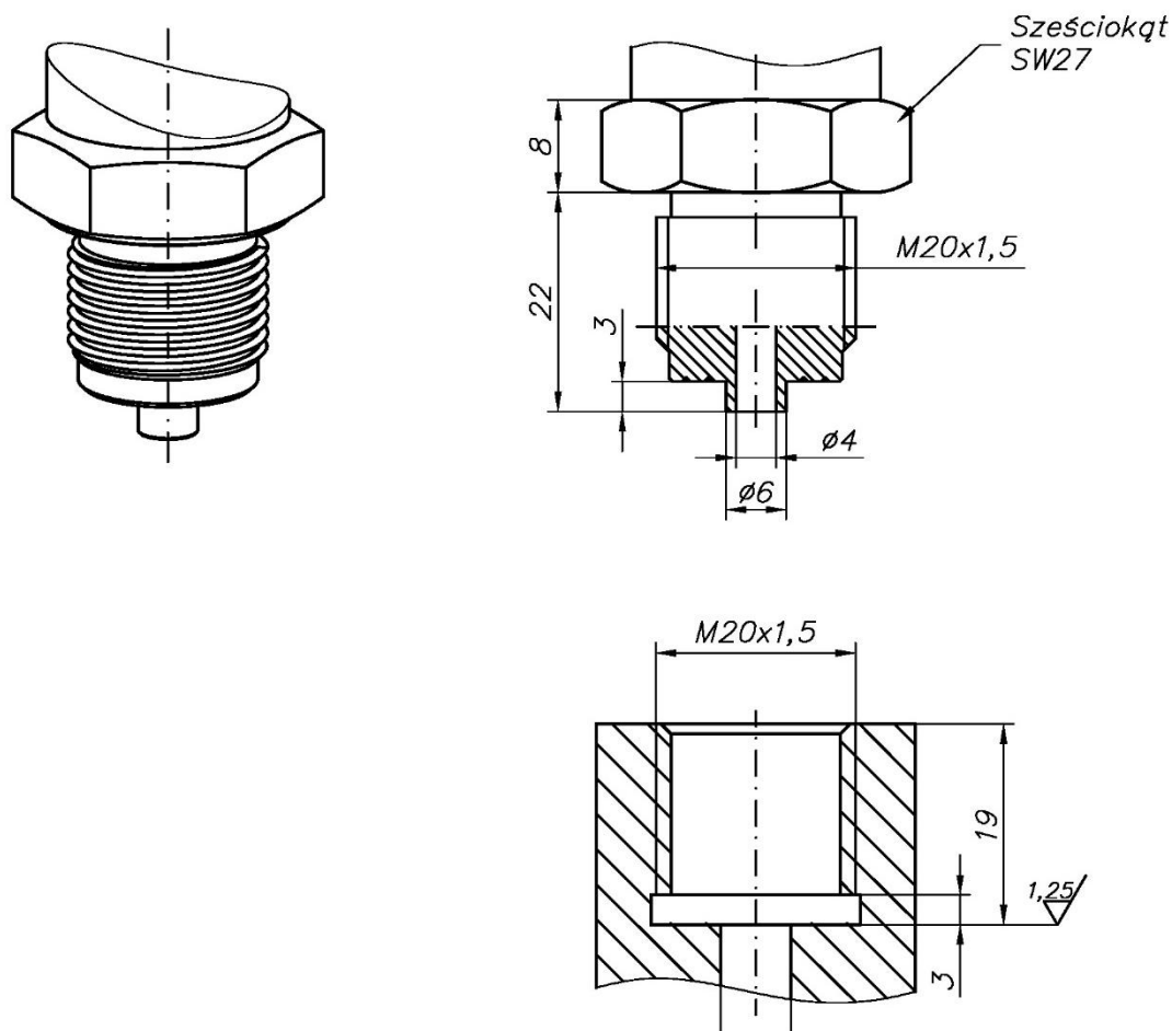
Rysunek 42. Przyłącze typu M (M20x1,5, \varnothing 4 ) z gniazdem.
