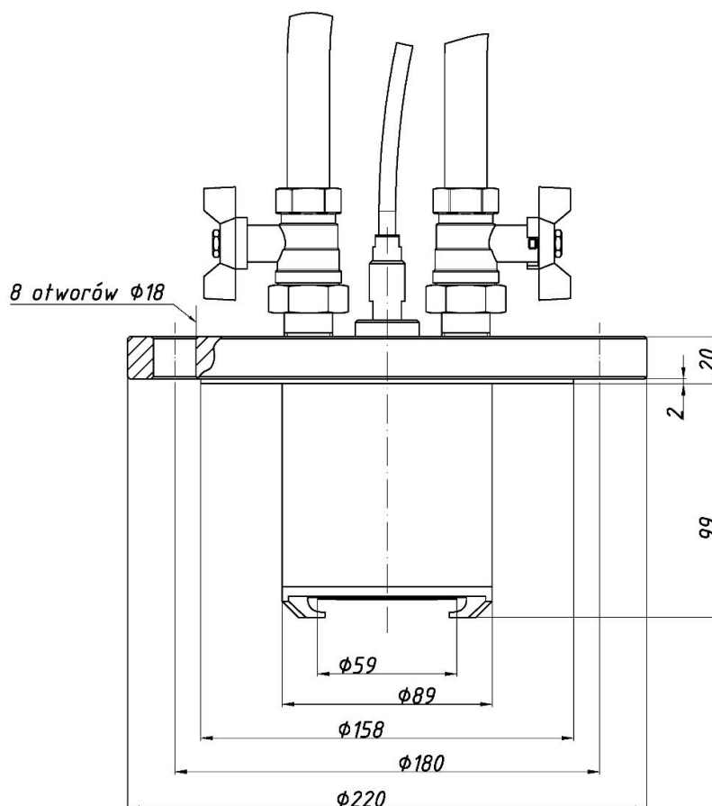
Rysunek 84. Separator S-TK-P z wbudowanym zespołem sflukiwania membrany - gabaryty.
