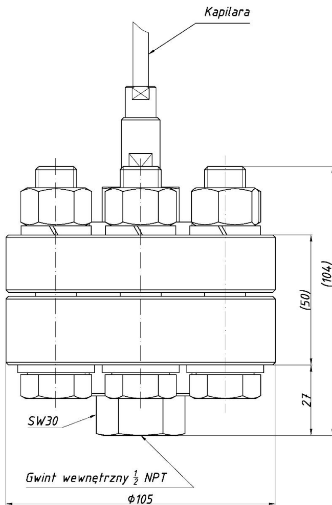
Rysunek 99. Separator S-Comp60MPa - gabaryty.
