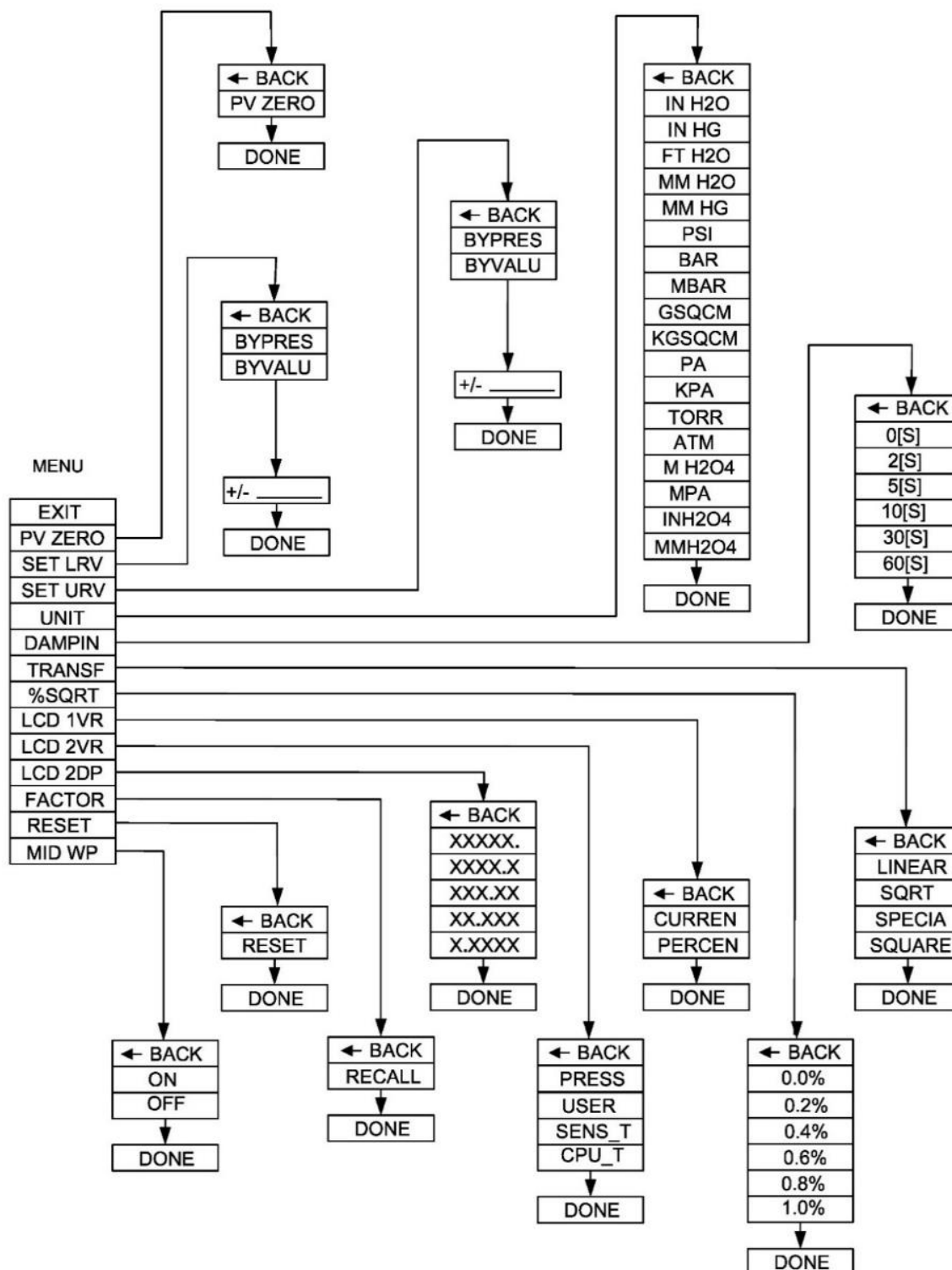
Rysunek 13. Struktura menu lokalnych nastaw przetwornika
