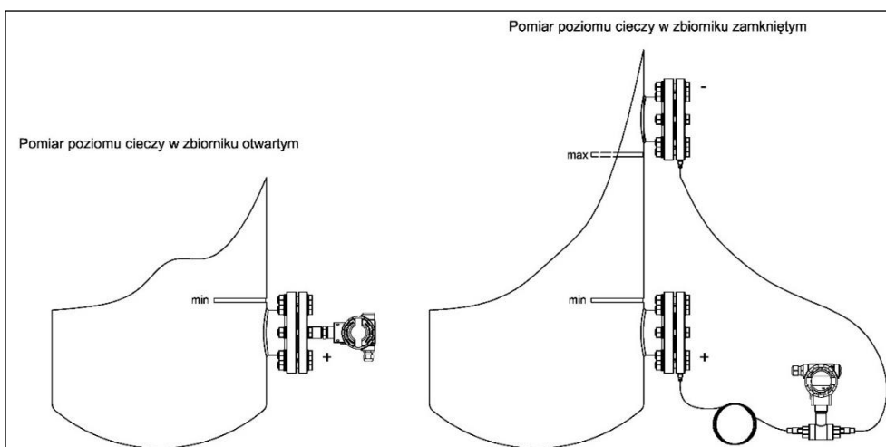
Rysunek 3. Przykłady montażu przetworników różnicy ciśnień
