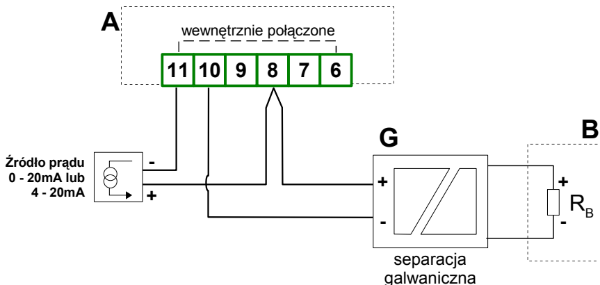
Rys. 4.12. Podłączenie przetwornika 2-przewodowego aktywnego z wyprowadzeniem sygnału prądowego do innego układu pomiarowego (np. sterownika PLC)
