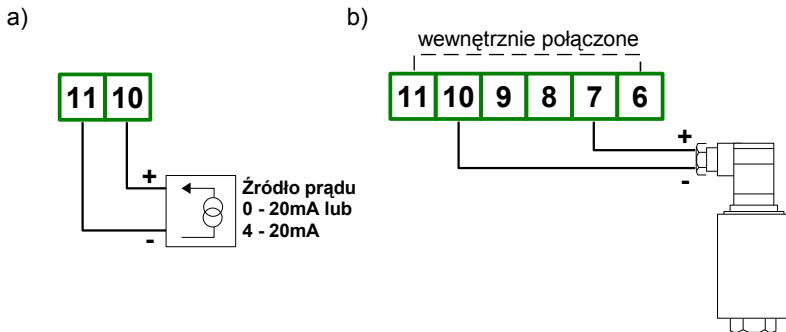
Rys. 4.11. Podłączenie przetwornika 2-przewodowego: a) aktywnego, b) pasywnego (wymagającego dodatkowego zasilania)
