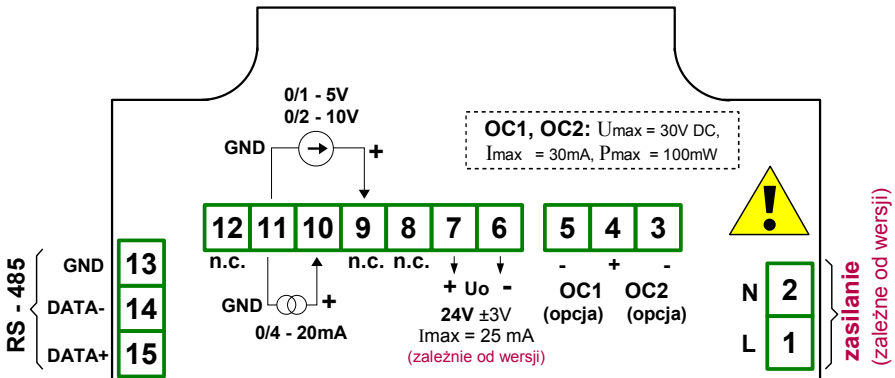
Rys. 4.4. Opis wyprowadzeń dla wersji z wyjściami OC
