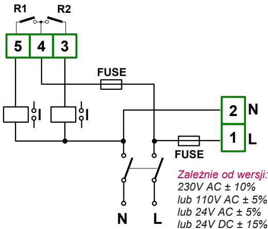
Rys. 4.8. Podłączenie zasilania oraz przekaźników sterujących obciążeniami
