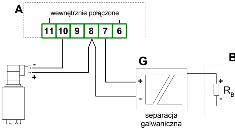
Rys. 4.13. Podłączenie przetwornika 2-przewodowego pasywnego z wyprowadzeniem sygnału prądowego do innego układu pomiarowego (np. sterownika PLC)
