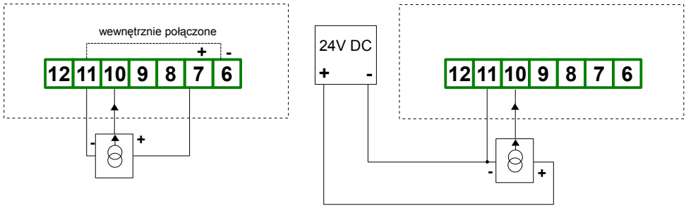
Rys. 4.6. Podłączenia przetworników prądowych 3 przewodowych
