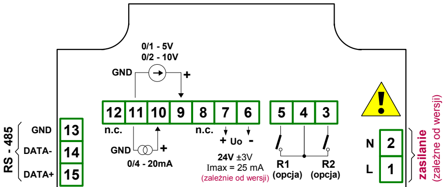
Rys. 4.3. Opis wyprowadzeń dla wersji z wyjściami przekaźnikowymi
