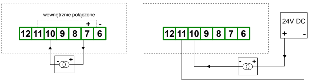
Rys. 4.5. Podłączenia przetworników prądowych 2 przewodowych
