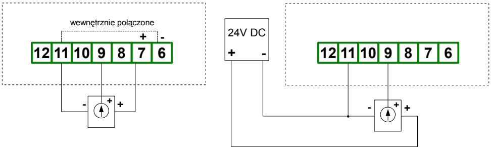
Rys. 4.7. Podłączenia przetworników napięciowych
