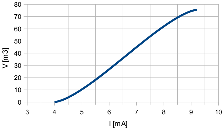
Rys. 9.7 Charakterystyka objętości zbiornika w zależności od prądu wejściowego z sondy poziomo cieczy w zbiorniku (dla zakresu 4÷20mA).
