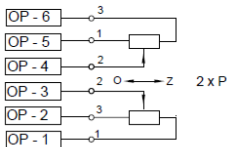
Wewnętrzne urządzenia siłownika z adresami połączeń
